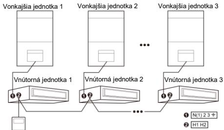
Obr. 4.6: Jeden ovládač ovláda súčasne niekoľko UNI SPLIT vnútorných jednotiek
