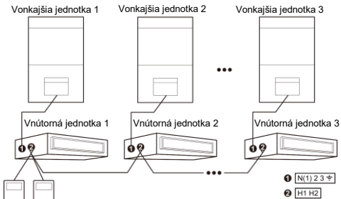
Obr. 4.7: Dva ovládače ovládajú súčasne niekoľko UNI SPLIT vnútorných jednotiek
