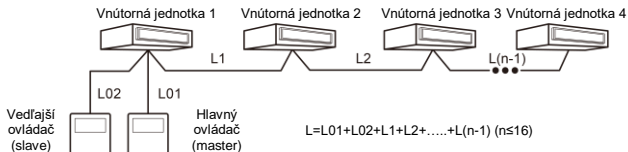
Obr. 4.3: Dĺžka komunikačného káblu
